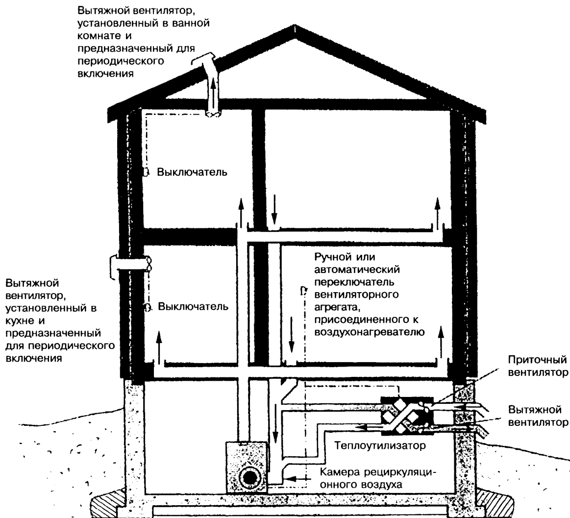
Рисунок 7.3 — Присоединение теплоутилизационного агрегата к камере подогрева воздуха
